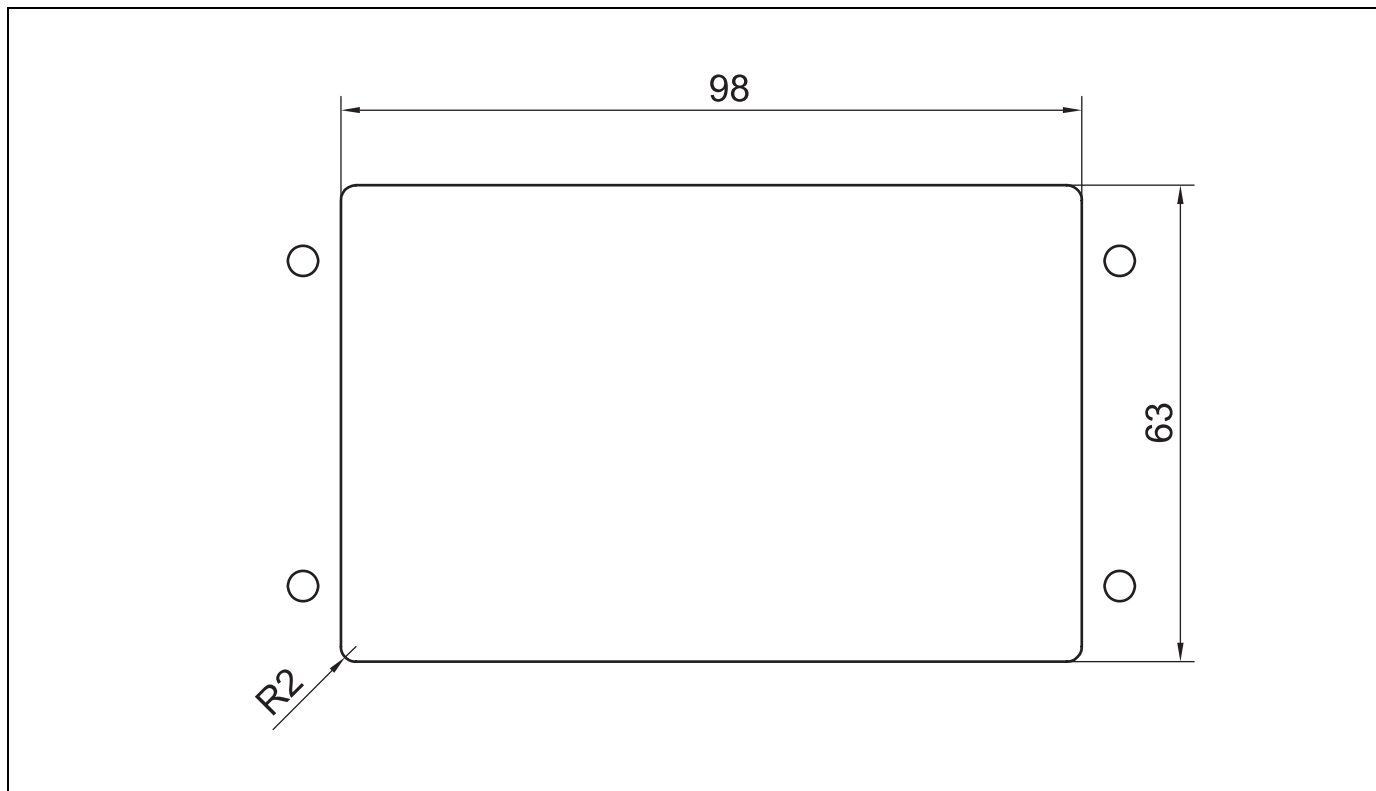
Рис.41: Шаблон для панели управления MC04/05
