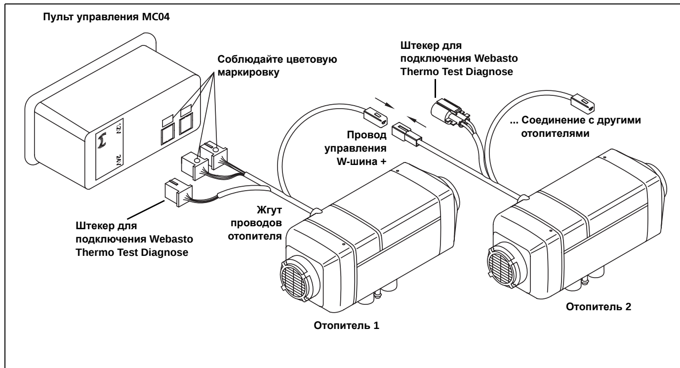
Рис.33: Схема электрических соединений Air Top Evo 3900 / 5500 AM с организацией системы главный/ведомый (вместо пульта управления возможно подключение таймера 1531 и/или температурного переключателя)
