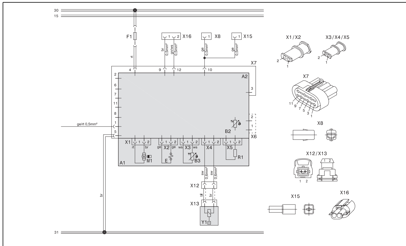
Рис.39: Электрическая схема Air Top Evo 3900 и Air Top Evo 5500 "ведомый отопитель (Slave)", 12V/24V дизель, экспликация приведена на стр. 137 и 138
