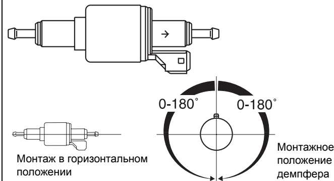
Рис.16: Дозирующий насос DP 30.2 Монтажное положение
